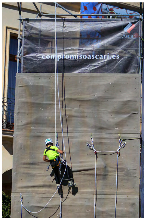
Detalles torres del Espeleódromo y vehículo de anclaje
